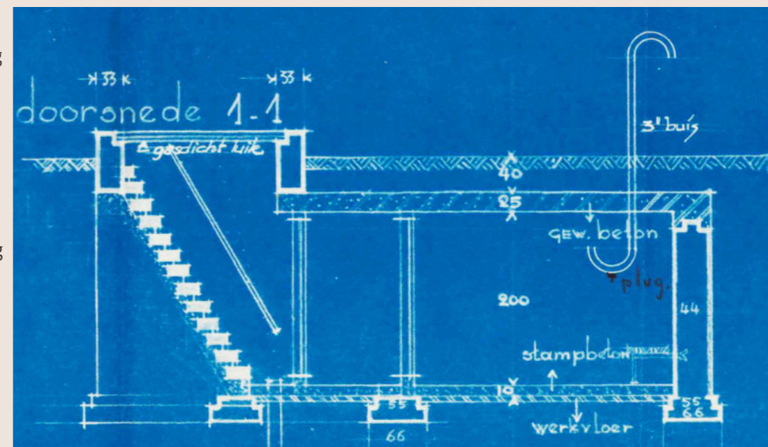
Uitsnede uit de bouwtekening voor de schuilkelder in de tuin van Julianalaan 86. Collectie Gelders archief
